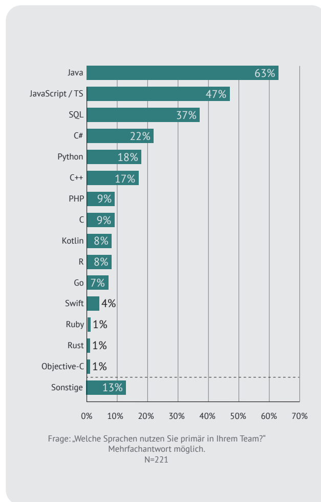
Abbildung 3: Überblick über die verwendeten Programmiersprachen
