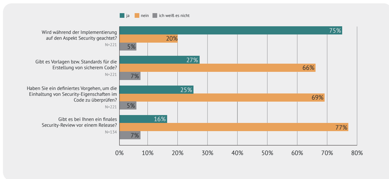
Abbildung 8: Berücksichtigung der Security in der Disziplin Implementierung und Test
